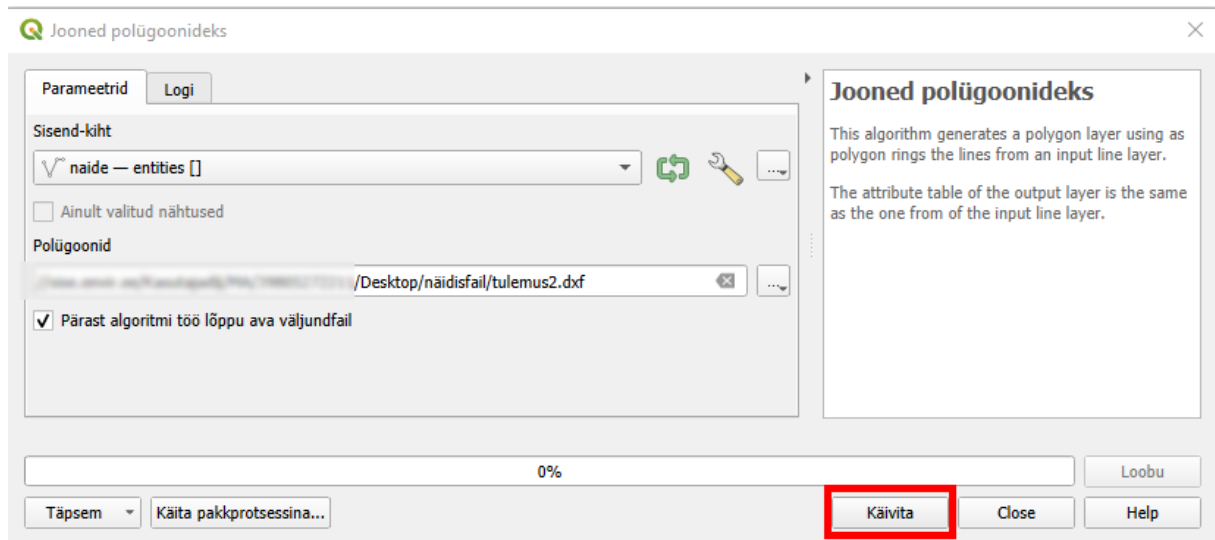
Joonis 9. „Jooned polügoonideks“ tööriista käivitamine.
